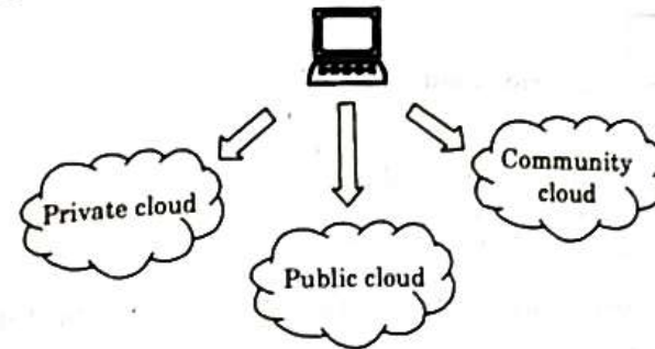
Fig. 3.10.1. Hybrid cloud.
