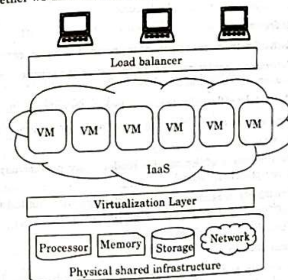
Fig. 3.14.1. IaaS.
