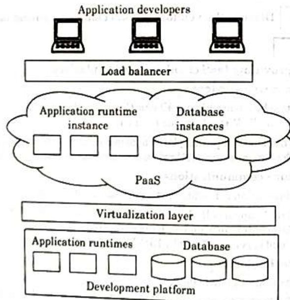
Fig-3.17.1. PaaS.
